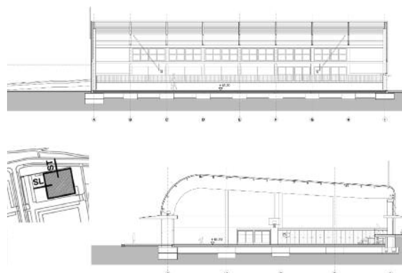
A l'esquerra, l'àmbit d'actuació per a l'ampliació de la zona esportiva. A la dreta, perfils nord i oest del nou pavelló.
